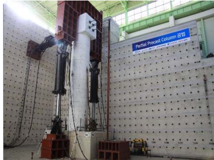
Precast 교각 성능실험
