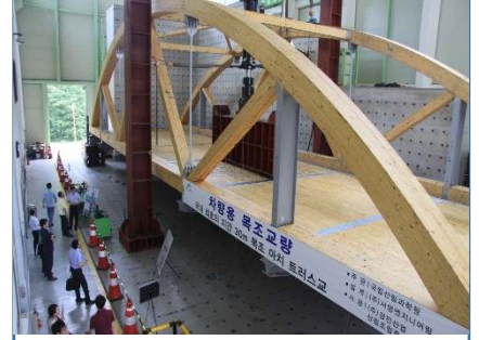
목조교량 성능실험
